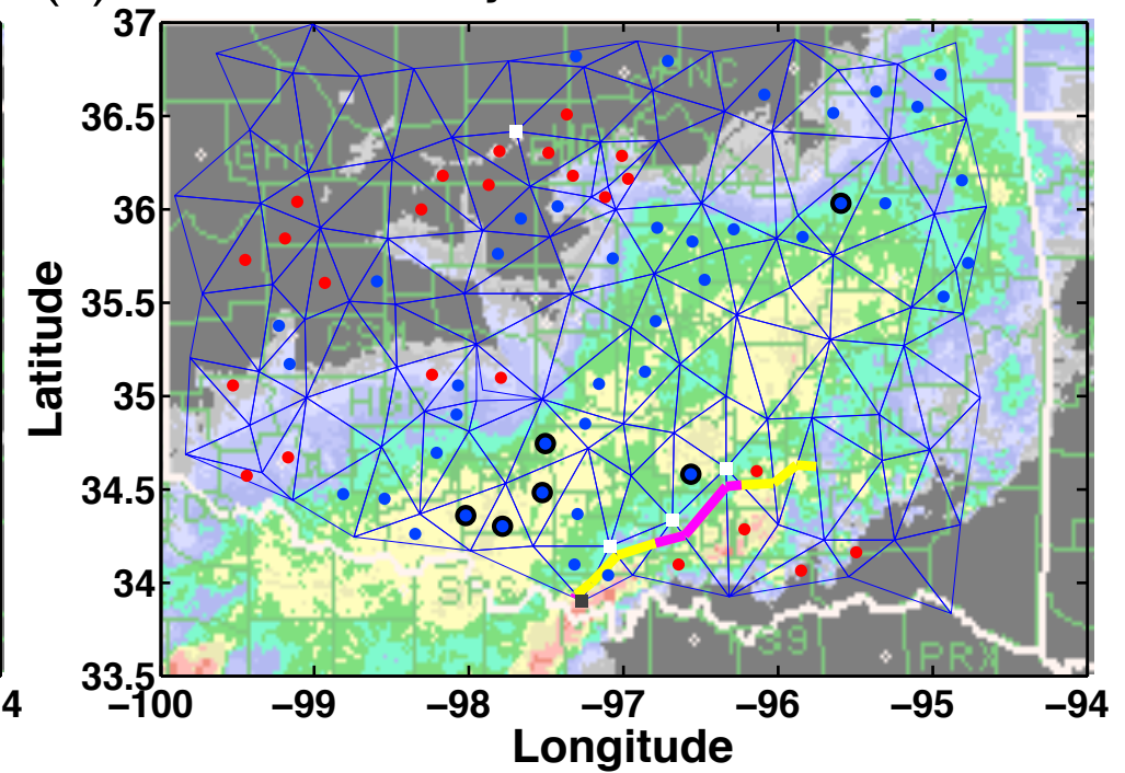
(d) Cold Pool Analysis 0430 UTC 16 June 2002
