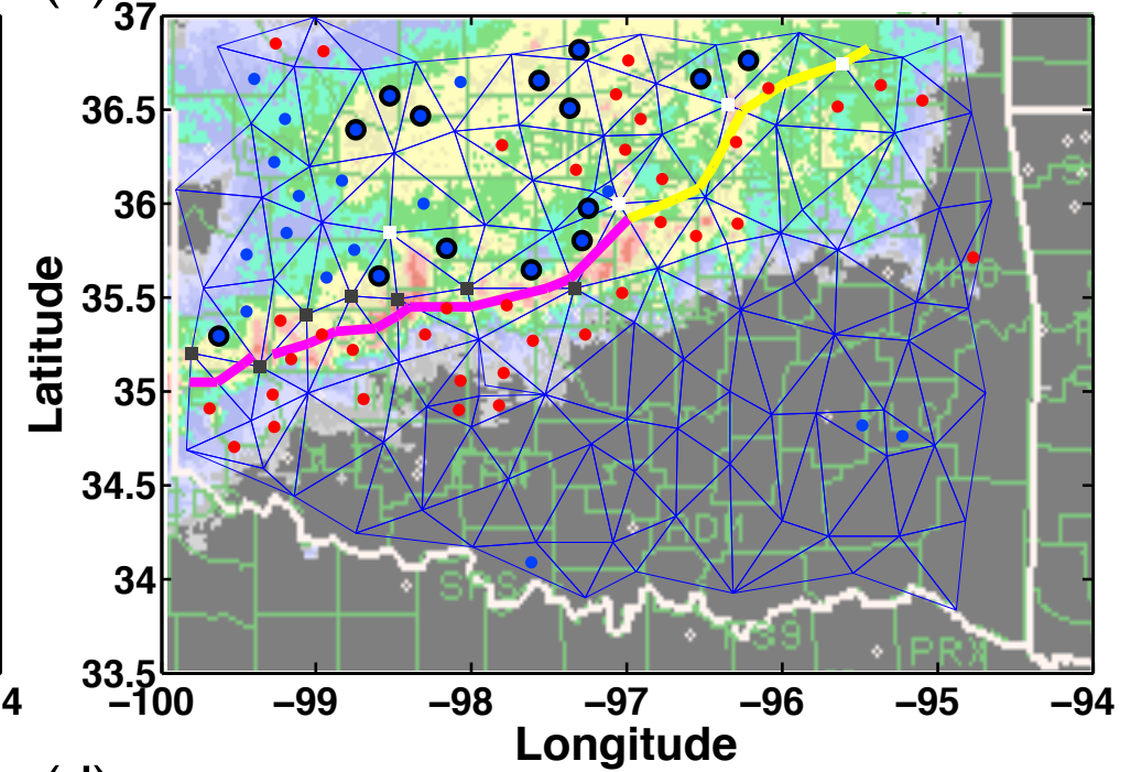
(d) Cold Pool Analysis 0430 UTC 16 June 2002
