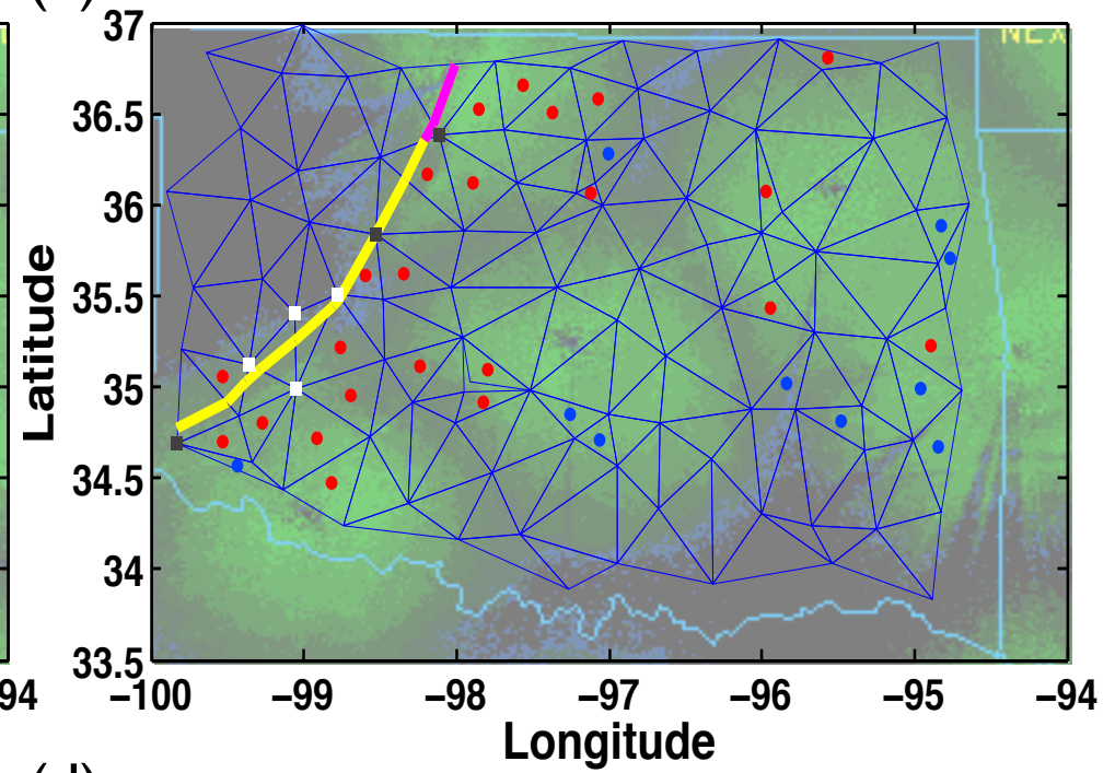
(d) Cold Pool Analysis 1500 UTC 30 April 2011
