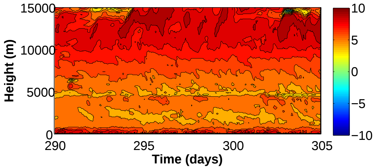
TABS lapse rate ( \text{K km}^{-1} ) NSA 1km
