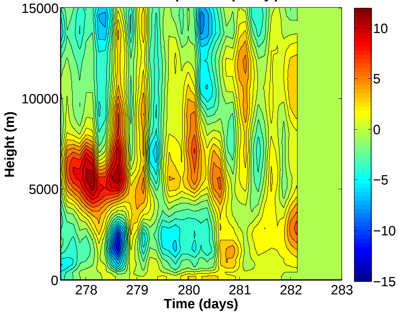
L.S. Horiz. Adv. Temp. Tend. ( \text{K day}^{-1} ) Revelle 1km
