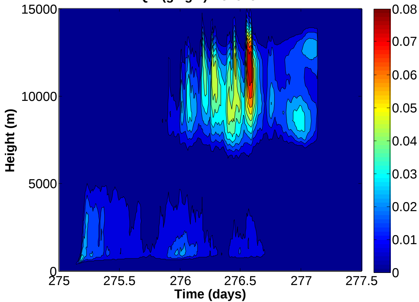
QN ( \text{g kg}^{-2} ) Revelle 1km
