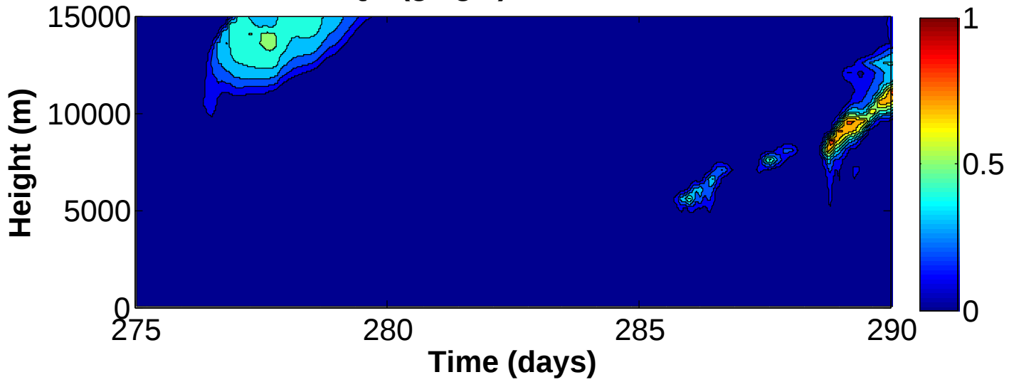
QN ( \text{g kg}^{-2} ) Revelle 1km
