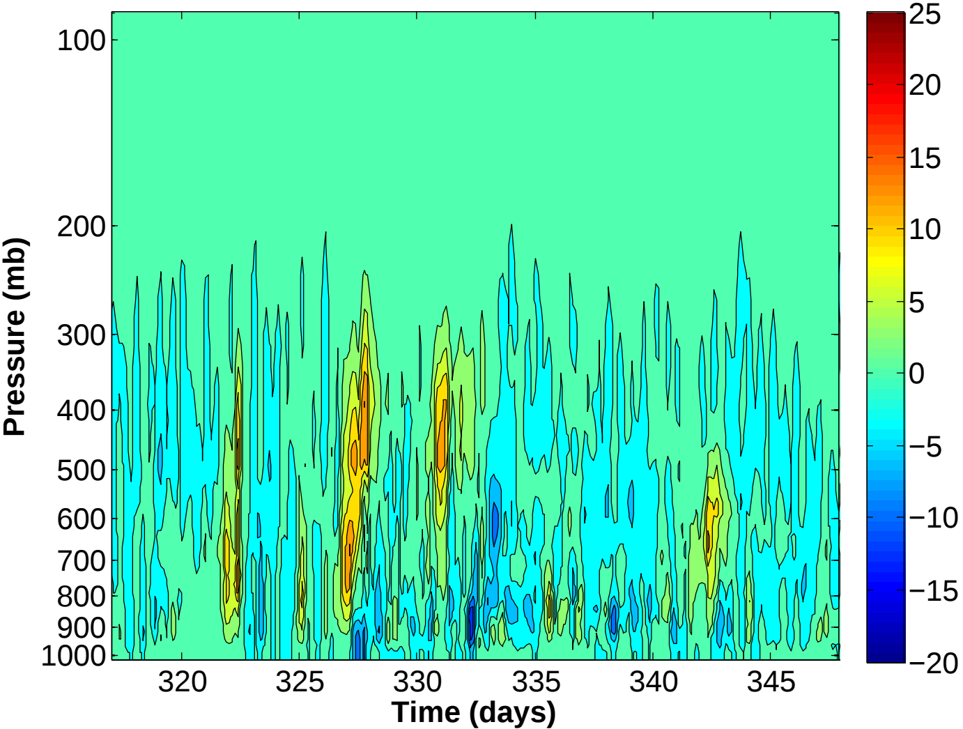
dat L.S. Adv. Moisture Tend. ( \text{g kg}^{-1} \text{ day}^{-1} ) Gan
