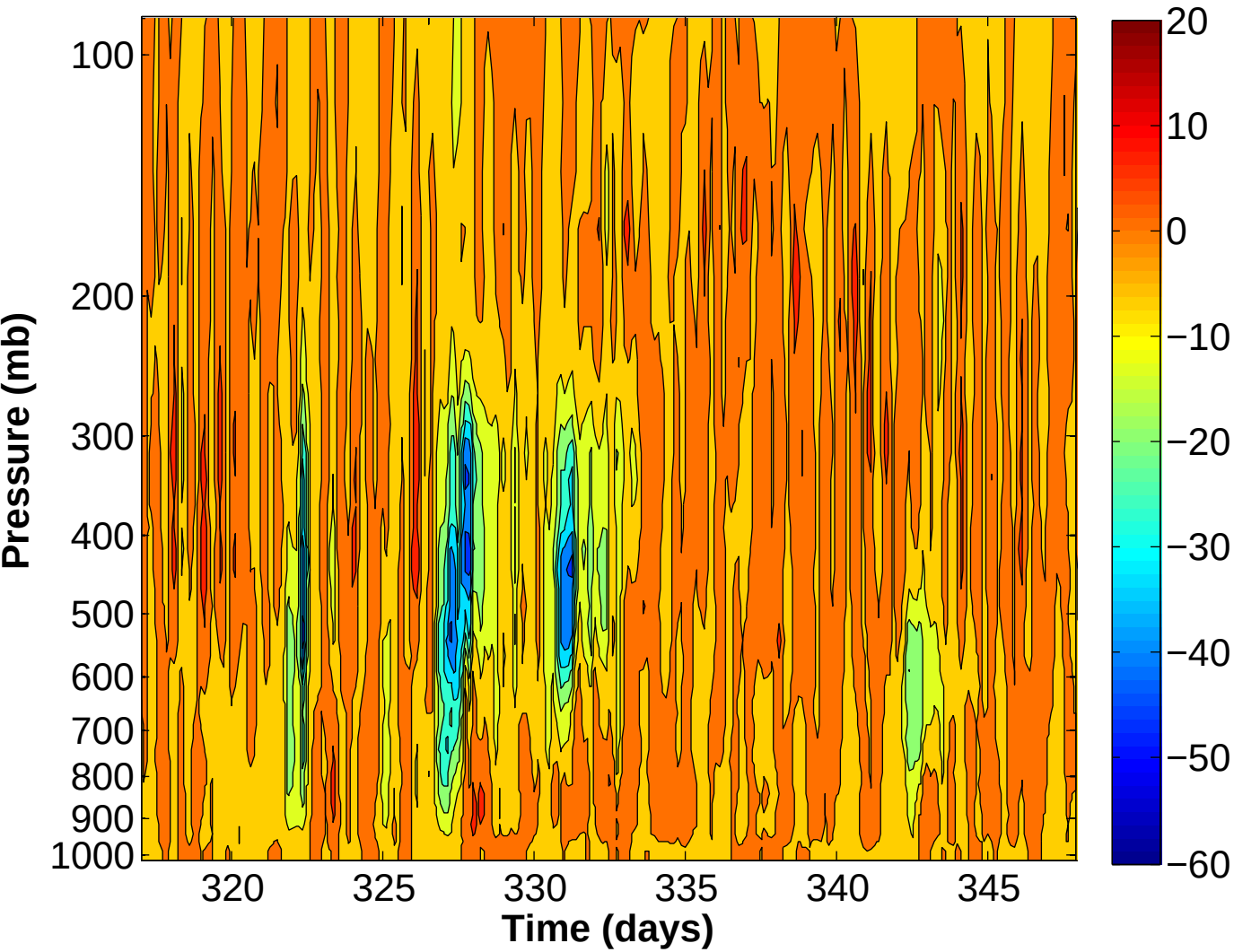
dat L.S. Adv. Temp. Tend. ( \text{K da}\bar{\text{y}}^{-1} ) Gan
