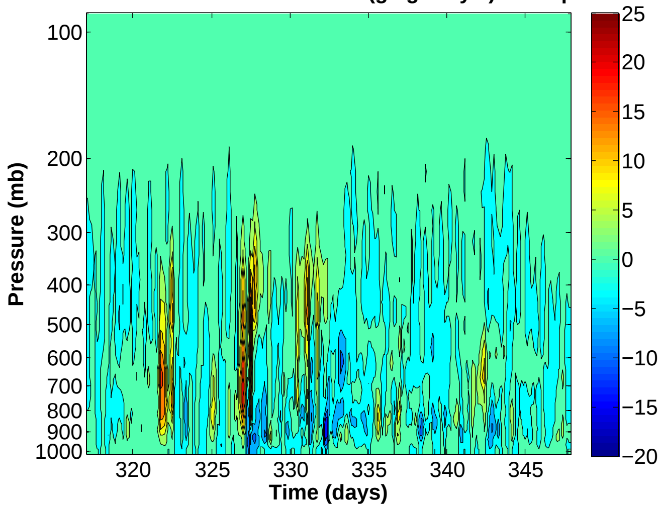
dat L.S. Adv. Moisture Tend. ( \text{g kg}^{-1} \text{ day}^{-1} ) Gan spol
