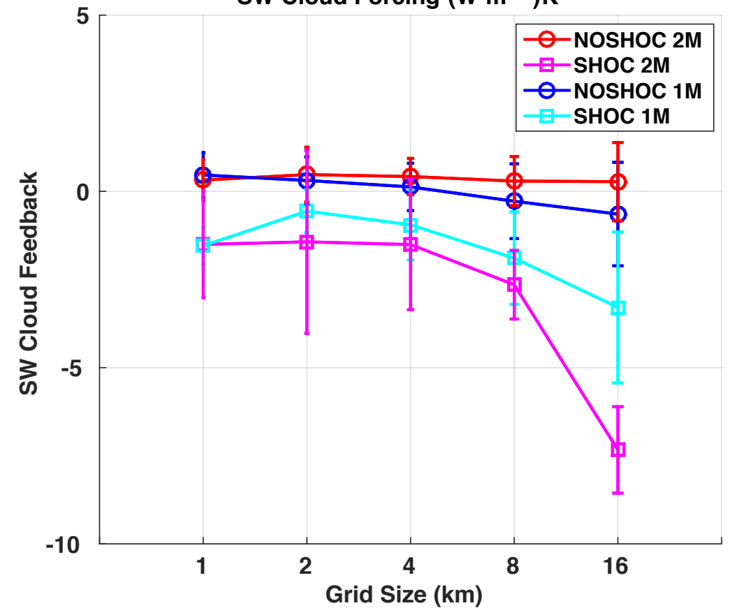
SW Cloud Forcing ( \text{W m}^{-2} \text{K}^{-1} )
