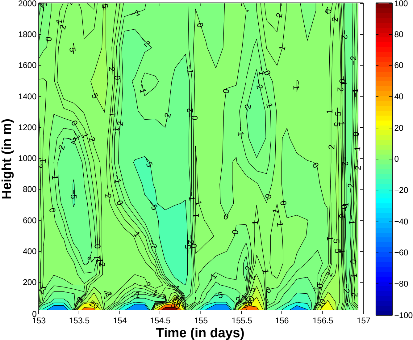
Run 204 (BL) Q1C: Apparent heat source Q1 – QR
