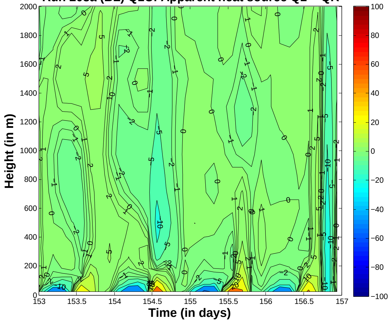
Run 208a (BL) Q1C: Apparent heat source Q1 – QR
