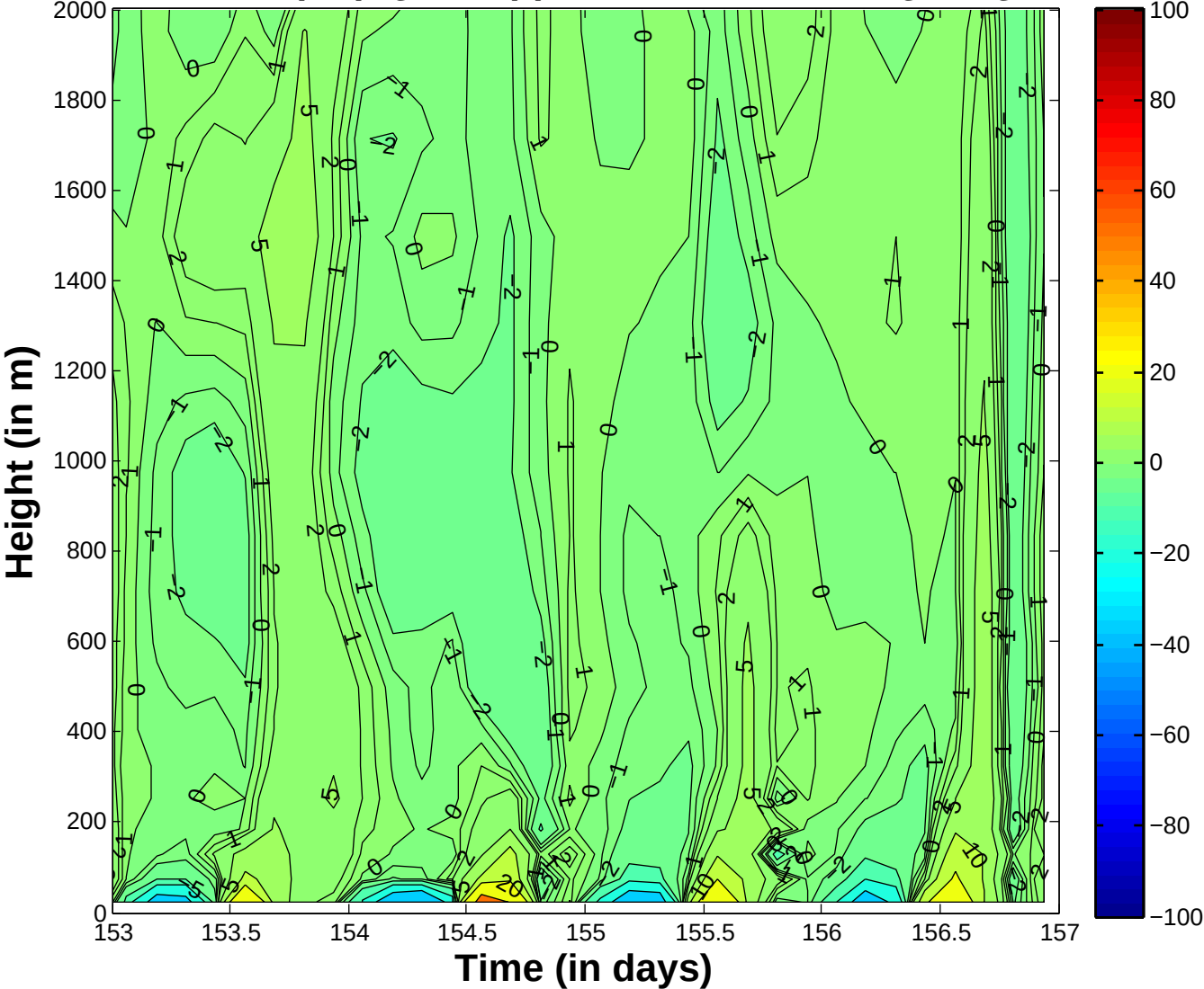
Run 304 (BL) Q1C: Apparent heat source Q1 – QR
