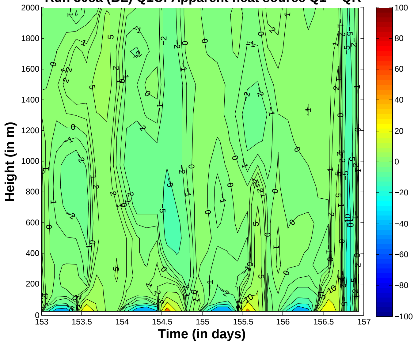
Run 308a (BL) Q1C: Apparent heat source Q1 – QR
