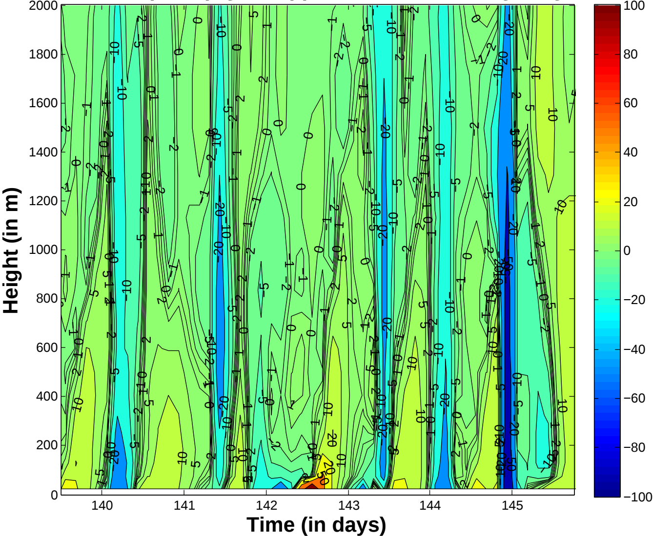
Run 204 (Conv) Q1C: Apparent heat source Q1 – QR
