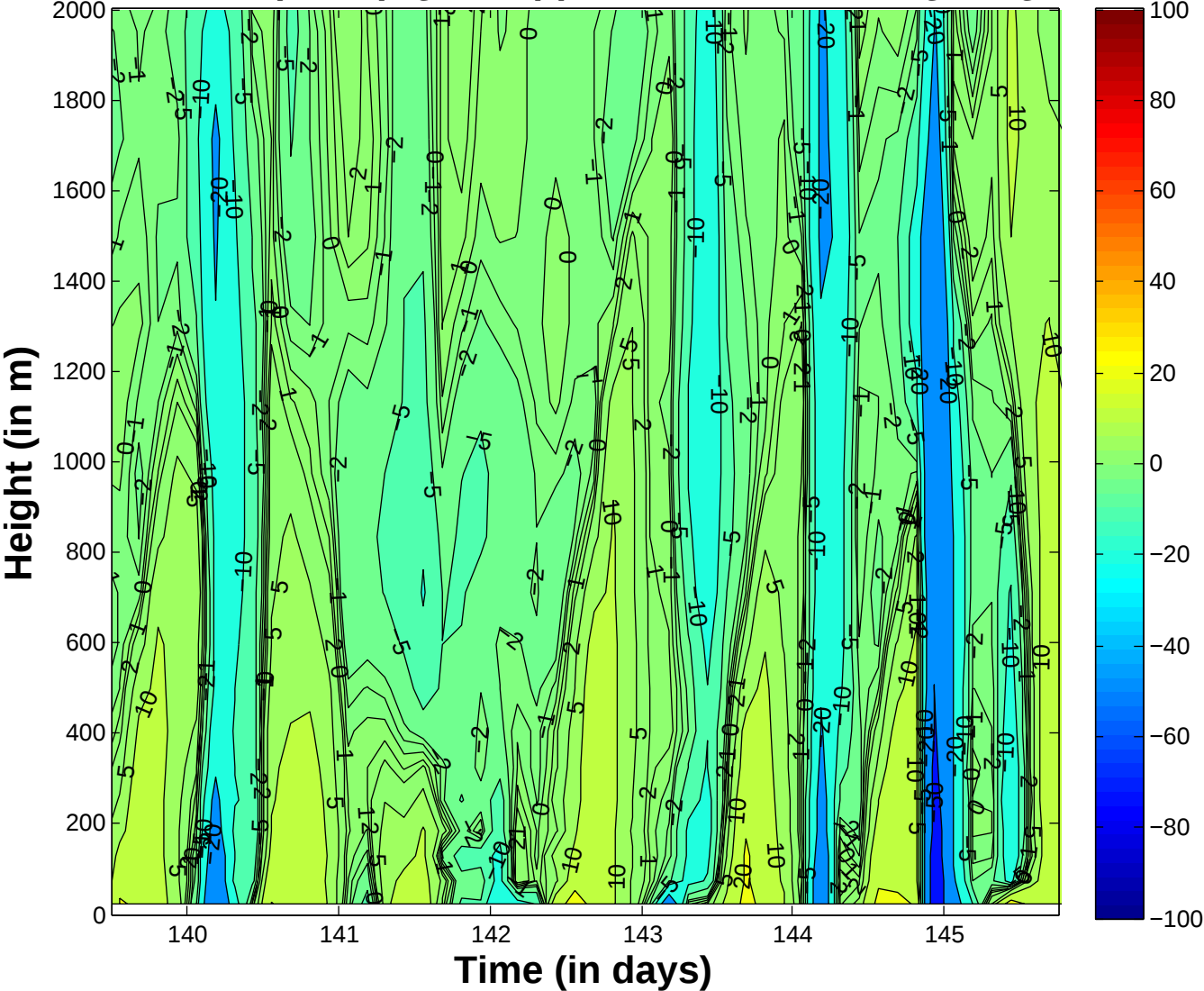
Run 304 (Conv) Q1C: Apparent heat source Q1 – QR
