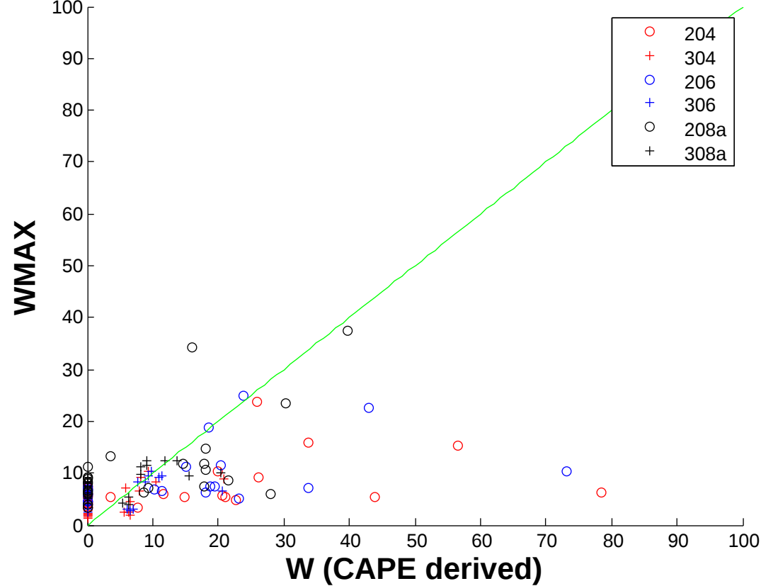
Day 153–156 WCAPE vs WMAX SHOC & Grid Comparisor
