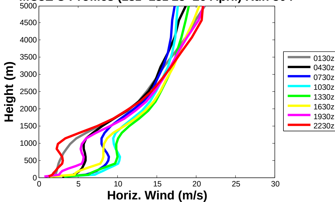
MC3E U Profiles (18z–18z 25–26 April) Run 304
