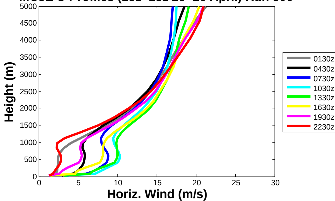
MC3E U Profiles (18z–18z 25–26 April) Run 306
