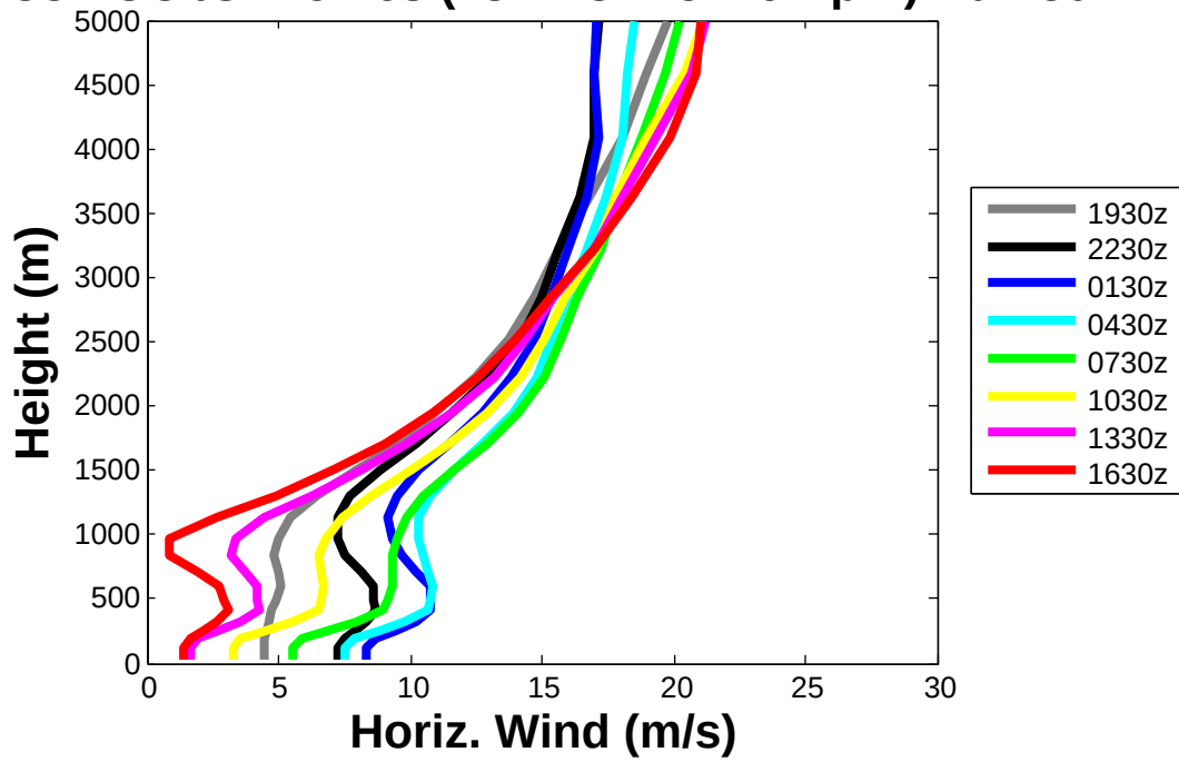
MC3E UObs Profiles (18z–18z 25–26 April) Run 304
