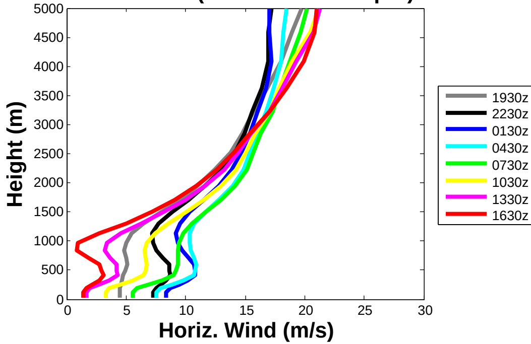
MC3E Uobs Profiles (18z–18z 25–26 April) Run 204
