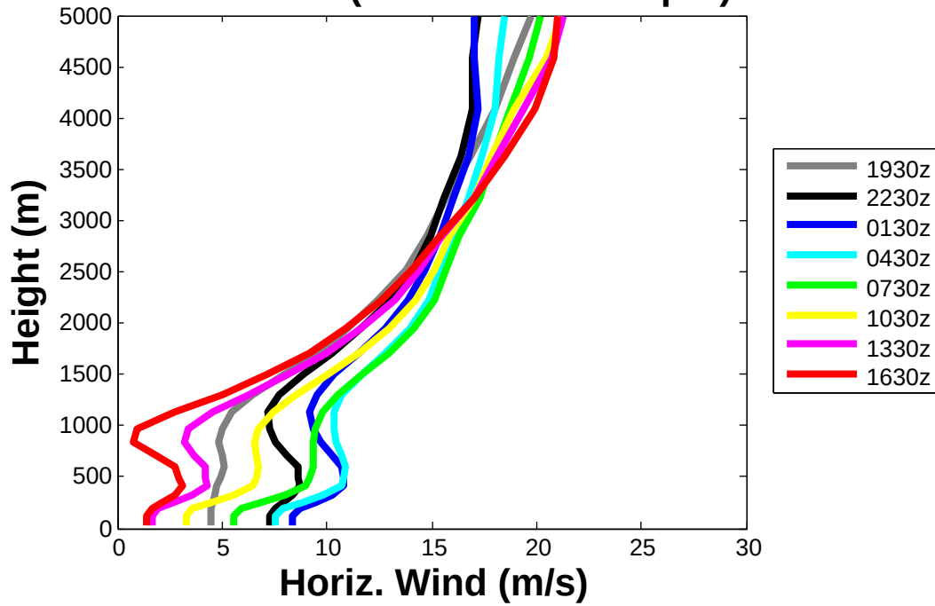
MC3E UObs Profiles (18z–18z 25–26 April) Run 206
