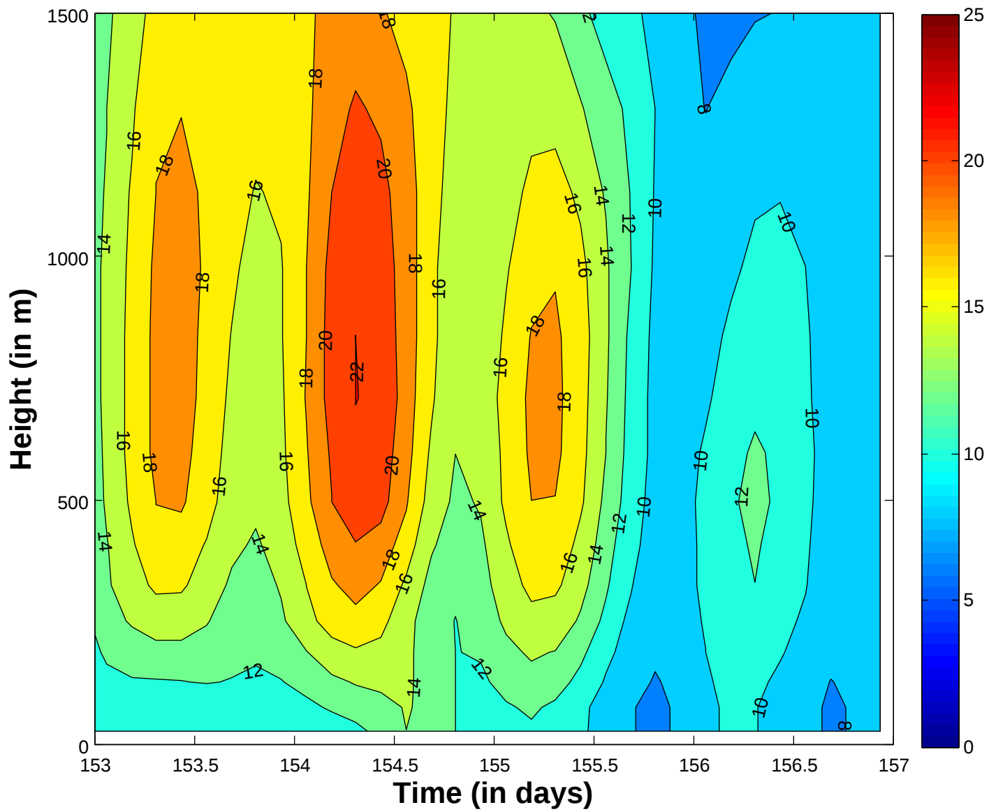
Run 306 Horiz. Wind Obs
