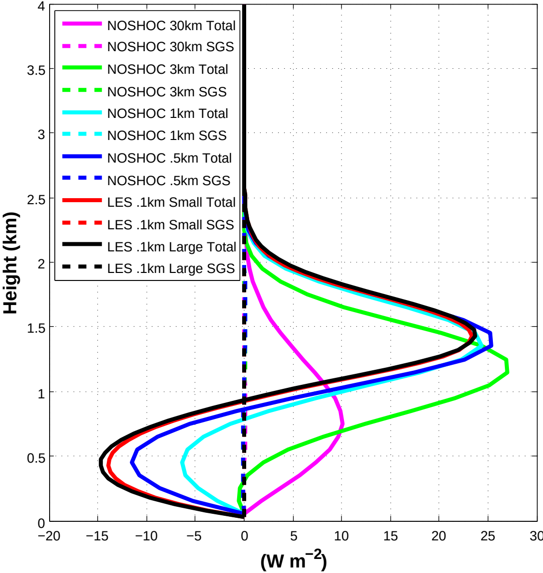
Precipitating-water turbulent flux (Full Phys.)
