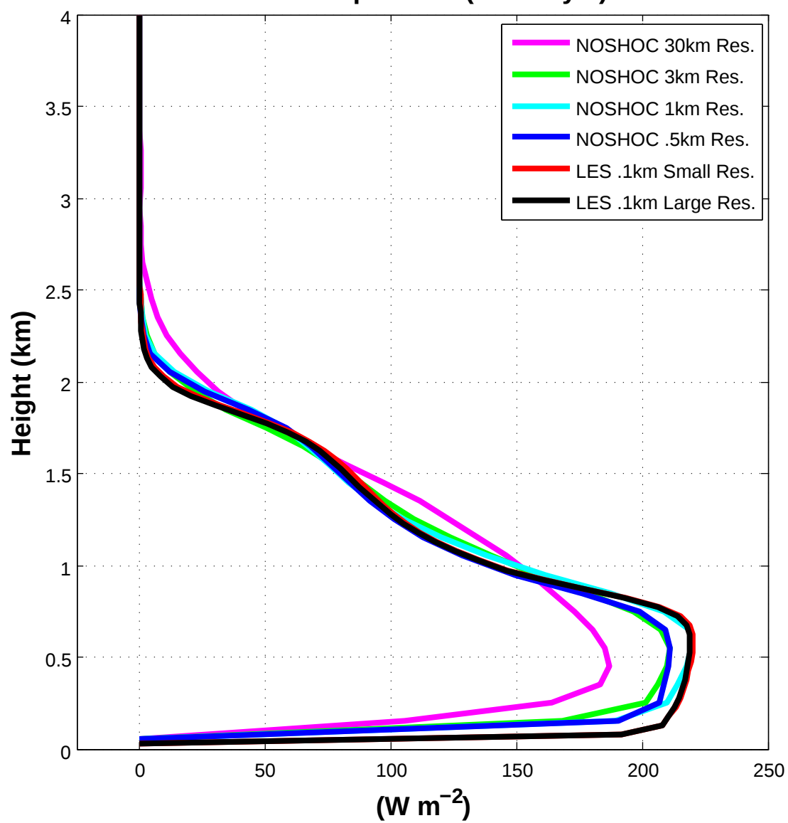
Water Vapor Flux (Full Phys.)
