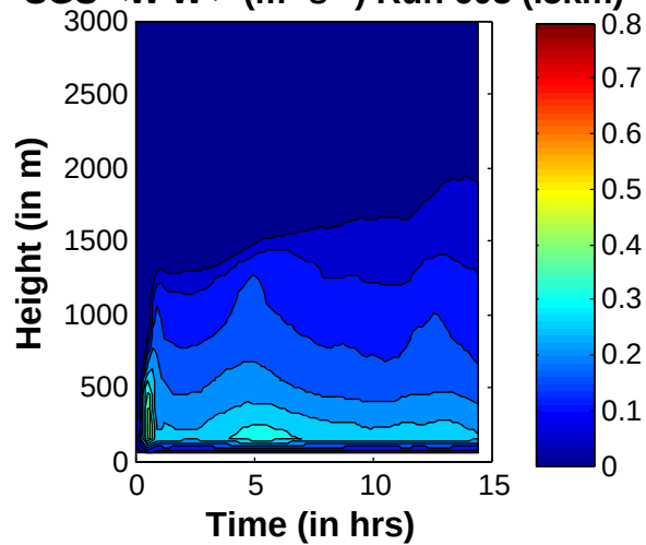
SGS \langle W'W' \rangle ( \text{m}^2 \text{s}^{-2} ) Run 603 (.5km)
