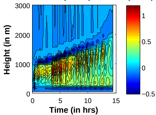
Total \langle W'W'W' \rangle ( \text{m}^3 \text{s}^{-3} ) Run 602 (1km)
