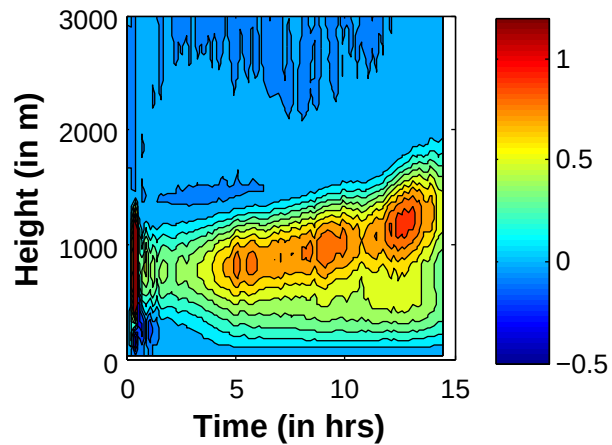
Total \langle W'W'W' \rangle ( \text{m}^3 \text{s}^{-3} ) Run 805b (.1km)
