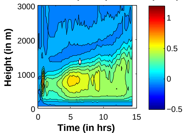
Total \langle W'W'W' \rangle ( \text{m}^3 \text{s}^{-3} ) Run 603 (.5km)
