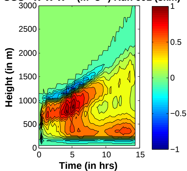
SGS \langle W'W'W' \rangle ( \text{m}^3 \text{s}^{-3} ) Run 601 (3km)
