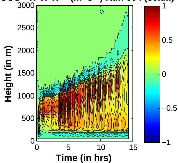
SGS \langle W'W'W' \rangle ( \text{m}^3 \text{s}^{-3} ) Run 604 (30km)
