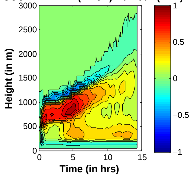
SGS \langle W'W'W' \rangle ( \text{m}^3 \text{s}^{-3} ) Run 602 (1km)
