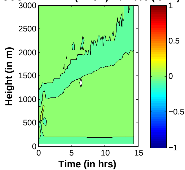
SGS \langle W'W'W' \rangle ( \text{m}^3 \text{s}^{-3} ) Run 603 (.5km)
