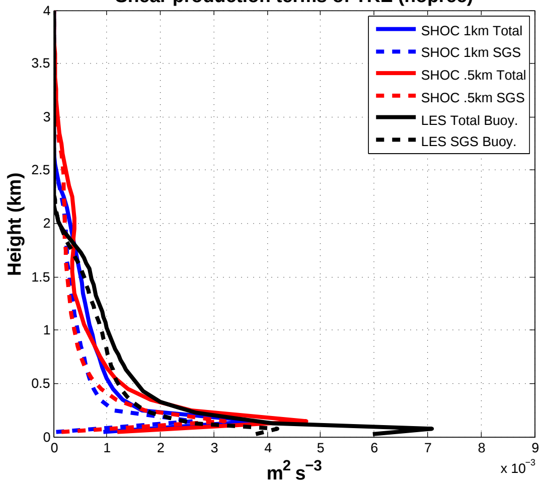
Shear production terms of TKE (noprec)
