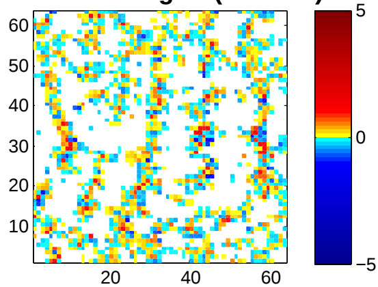
Mean w 1km grid (z=775m)
