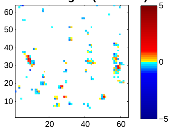
Mean w 1km grid (z=2275m)
