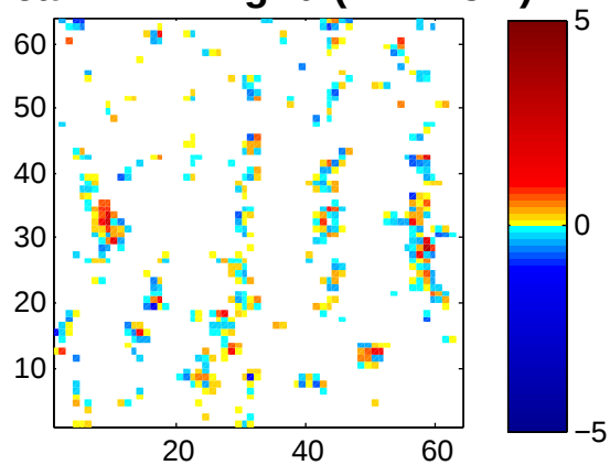
Mean w 1km grid (z=1775m)
