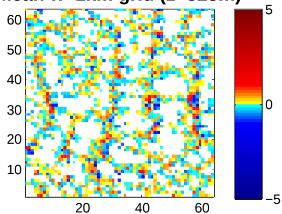
Mean w 1km grid (z=525m)
