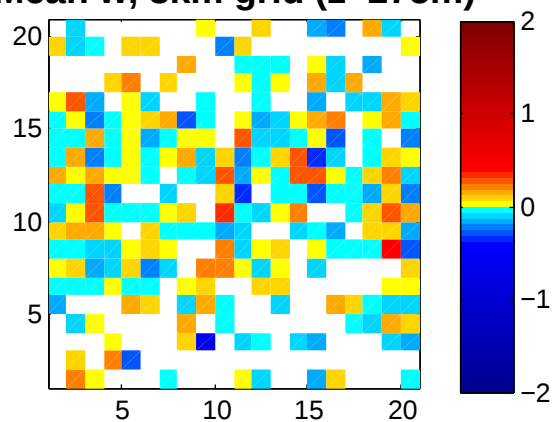
Mean w, 3km grid (z=275m)
