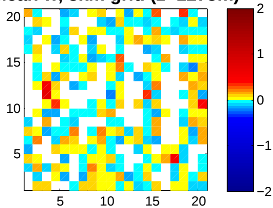
Mean w, 3km grid (z=1275m)
