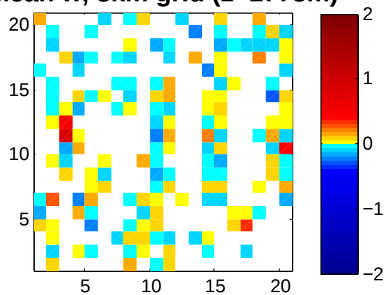
Mean w, 3km grid (z=1775m)
