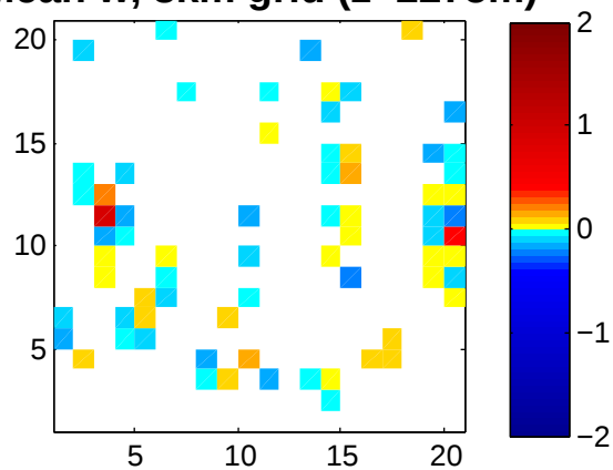
Mean w, 3km grid (z=2275m)
