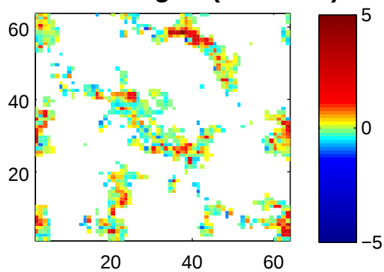
Mean w 1km grid (z=1525m)
