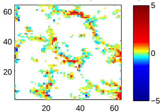
Mean w 1km grid (z=1025m)
