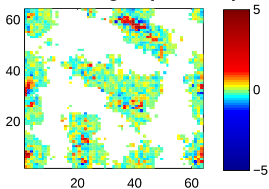
Mean w 1km grid (z=2525m)
