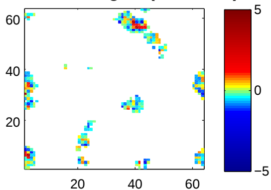
Mean w 1km grid (z=3025m)
