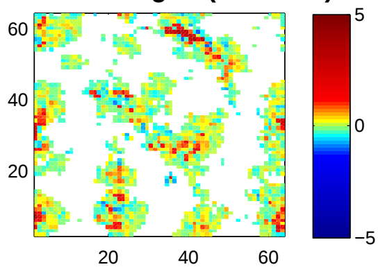
Mean w 1km grid (z=2025m)
