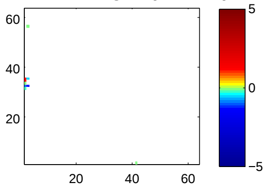
Mean w 1km grid (z=525m)
