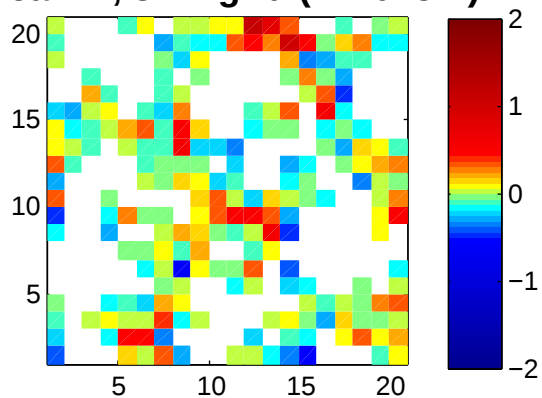
Mean w, 3km grid (z=1025m)
