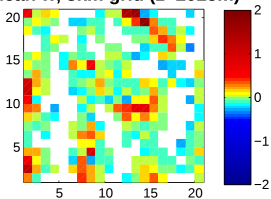
Mean w, 3km grid (z=2025m)
