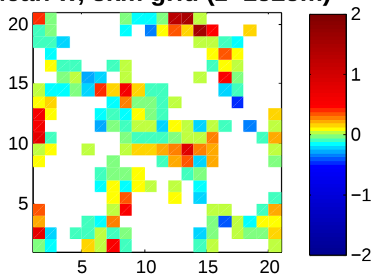
Mean w, 3km grid (z=1525m)
