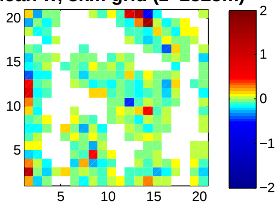
Mean w, 3km grid (z=2525m)
