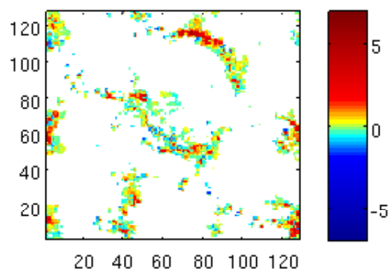
Mean w, .5km grid (z=1525m)
