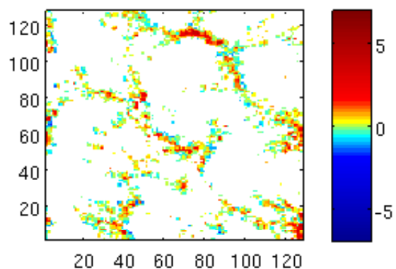
Mean w, .5km grid (z=1025m)
