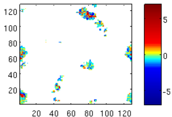
Mean w, .5km grid (z=3025m)
