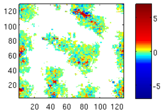
Mean w, .5km grid (z=2525m)
