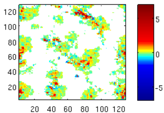
Mean w, .5km grid (z=2025m)
