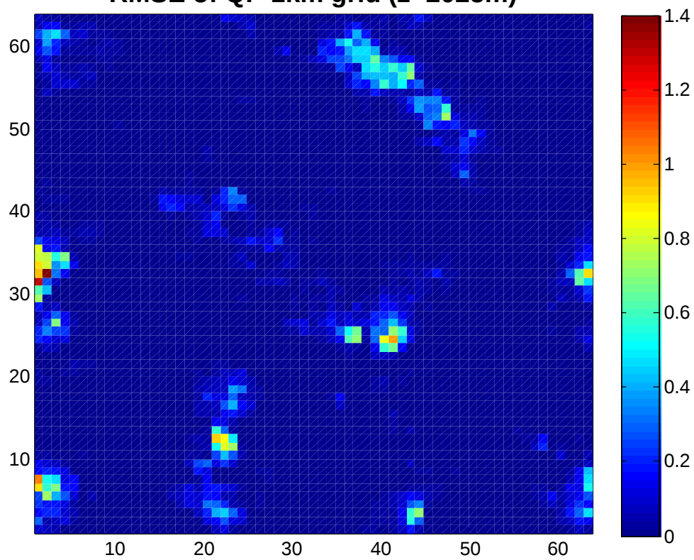
RMSE of QP 1km grid (z=2025m)
