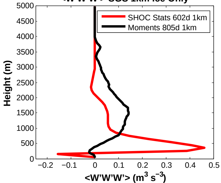
<W'W'W'> SGS 1km Ice Only
