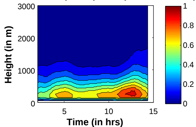
Total \langle W'W' \rangle ( \text{m}^2 \text{s}^{-2} ) 805d (LES ice)
