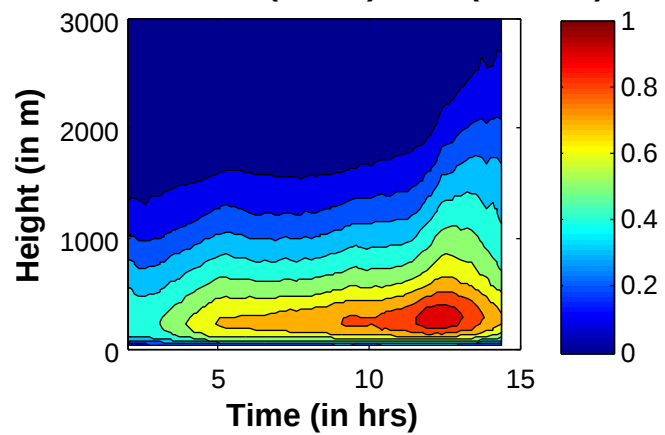
Total \langle W'W' \rangle ( \text{m}^2 \text{s}^{-2} ) 805d (LES ice)
