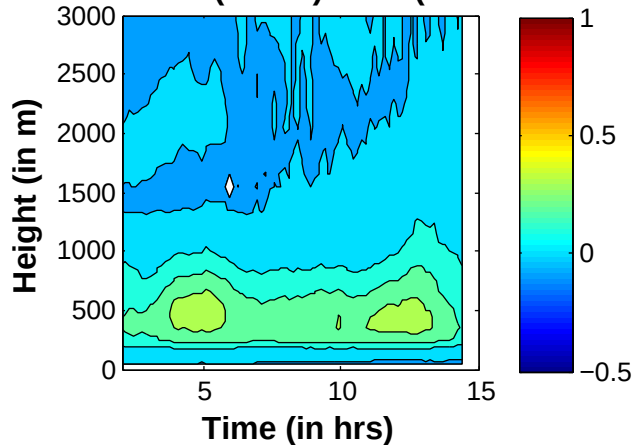
Total \langle W'W'W' \rangle ( \text{m}^2 \text{s}^{-2} ) 805d (LES ice)
