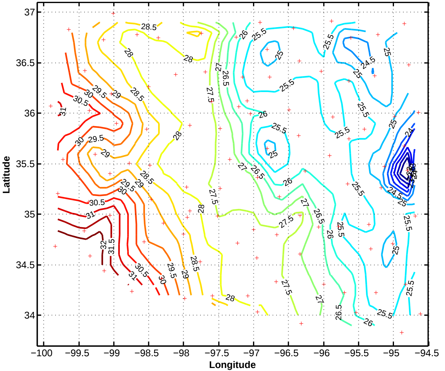
6/12/97 0000z Mesonet Temperature (Celsius)
