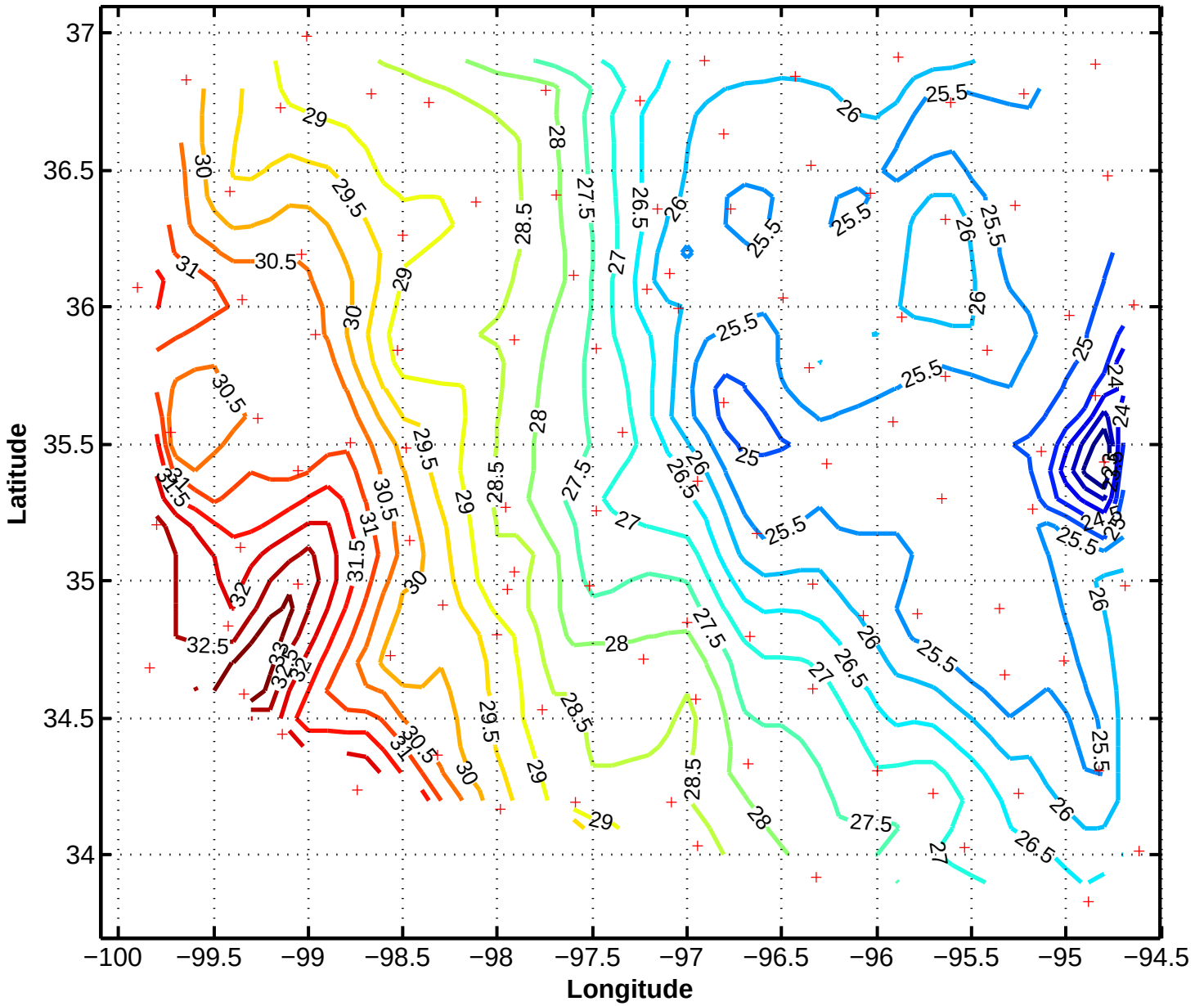
6/11/97 2300z Mesonet Temperature (Celsius)
